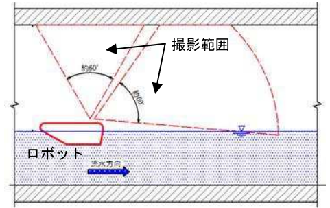
図-6 撮影範囲縦断面図
