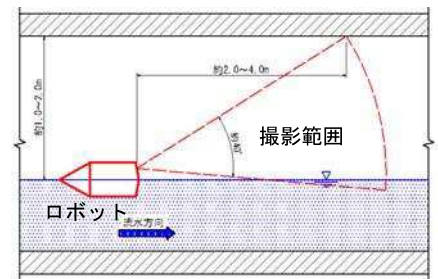
図-2 撮影範囲縦断面図
