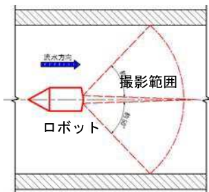
図-1 撮影範囲平面図
