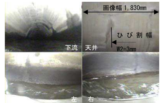
図-8 撮影画像(例)
