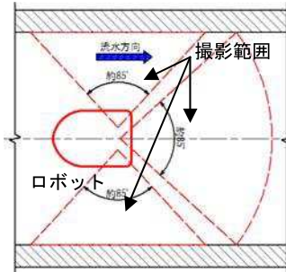
図-5 撮影範囲平面図
