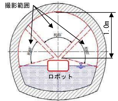
図-7 撮影範囲横断面図
